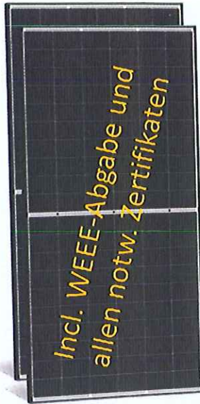
Abb. von oben: Hoymiles HM-300, DEYE SUN-M600 G3-EU 600 W mit WLAN, links zwei PV-Module mit 380 Wp
